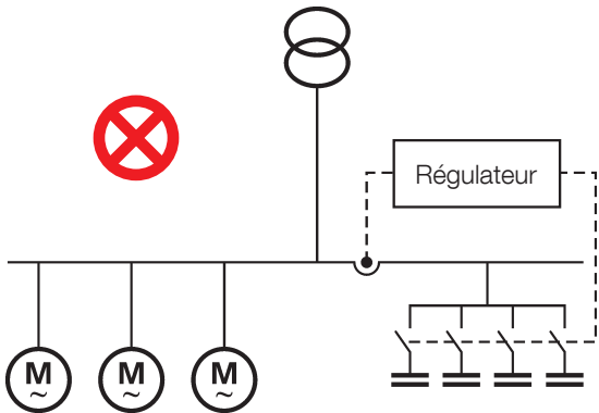
Fig. 3 : Incorrecte. Le transformateur ne mesure que le courant des condensateurs qui sera initialement de zéro, empêchant le fonctionnement du système. Alarme «Sous-intensité»
