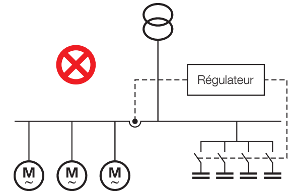
Fig. 2 : Incorrecte. Le transformateur ne mesure que le courant des charges de l’installation. Ni la régulation, ni la mise en service automatique ne peuvent fonctionner.
