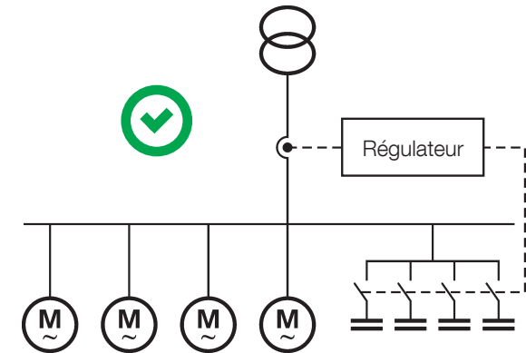
Fig. 1 :Correcte. Le transformateur mesure le courant des charges de l’installation et des condensateurs
