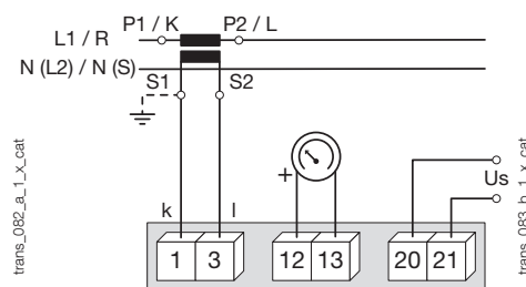
Aansluiting met 1 stroomtransfo en U_s
