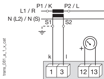
Aansluiting met 1 stroomtransfo zonder U_s
