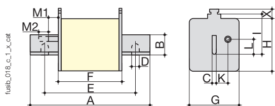
Afmetingen volgens IEC 60269-2-1
