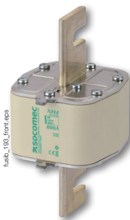
Zekering aM, NH4 van 315 tot 1250 A
