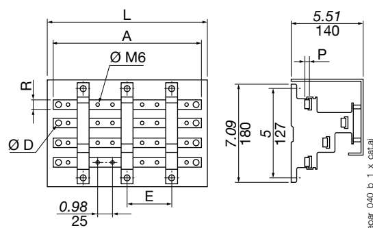
Répartiteur en escalier, avec trous taraudés, encliquetable sur rail DIN symétrique. Monté en usine et livré sans capot de protection.
