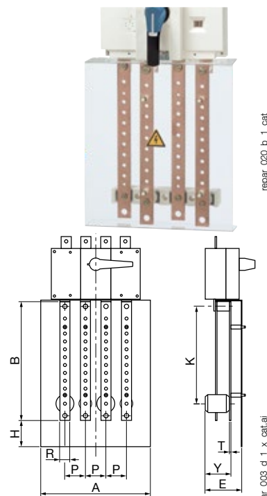
Répartiteur avec connexion par cosses, protection frontale contre les contacts fortuits (appareil de coupure non fourni).
