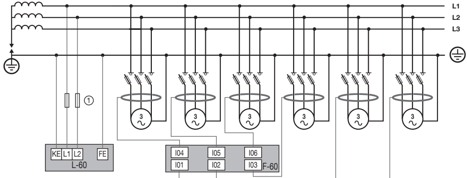
3AC / IMD + IFL
