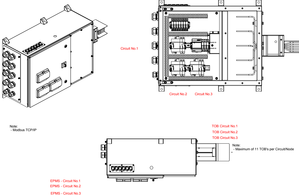
Fig 15. Coffret de dérivation de tête - multiples systèmes DIRIS Digiware en parallèle
